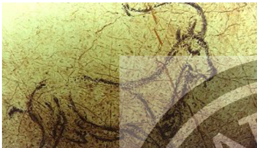
Eine Höhlenmalerei.
